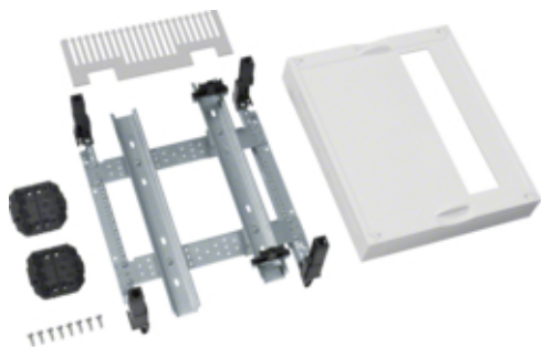
Блок Univers, 1 верт.шина TS35 для клемних колодок + 1х13мод., 300х250мм
