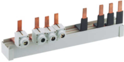
Шина для вимикачі в HІ...R
