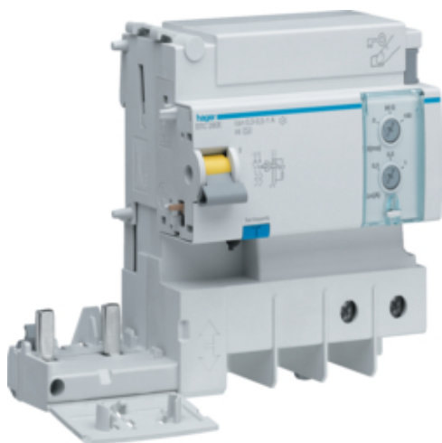
Блок ПЗВ 2-пол., In=125A, 0,3-0,5-1A, AC
