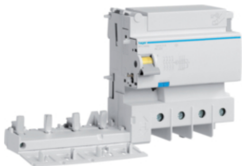
Блок ПЗВ 4-пол., In=125A, 300mA, AC
