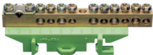
Клема захисна з тримачем 1x25+5x16+5x10мм 2
