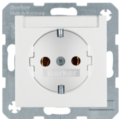
Розетка з з/к з полемд/надпису, пол.бі лизна, 16A/250В S.1
