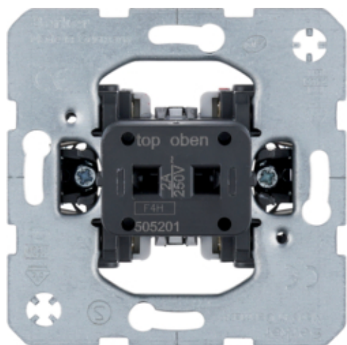
Кнопочний вимикач hotelcard, 1НВ+1НЗ, 2А/250В
