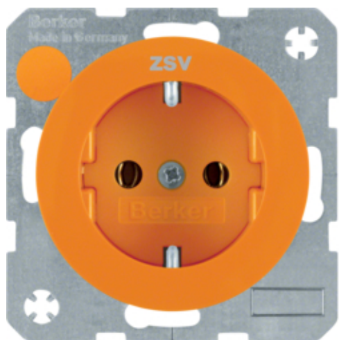
Розетка з з/к червона з надписом ZSV, 16A/250В, R.1/R.3
