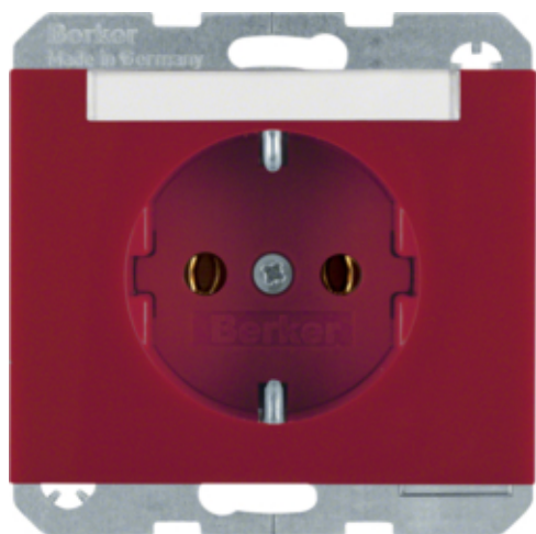
Розетка з з/к з полем д/надпису, червона, 16A/250V K.1
