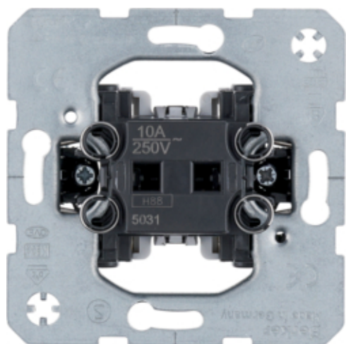
Кнопка 1-клатві шна 1НВ (механі зм) 10А/250В
