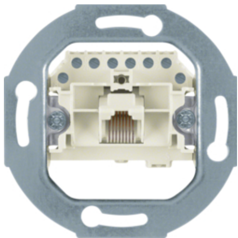
Розетка UAE 8-полкџн., Кат.3
