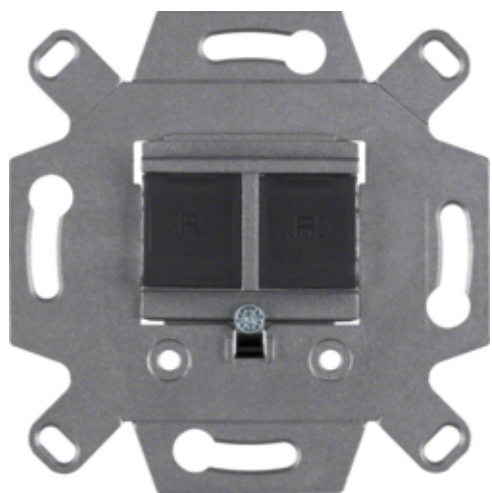
Розетка UAE 8/8-полкѡн. екранована, Кат.6A iso
