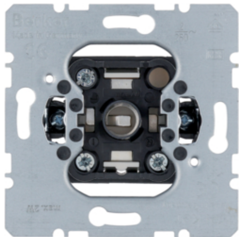
Нажимна кнопка та світловий сигнал E10
