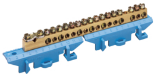
Клема нейтральна з тримачем 1x25+8x16+8x10мм 2
