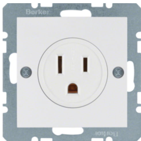
Розетка без з/к Євро-американська, пол.бі лизна, 16A/250B S.1
