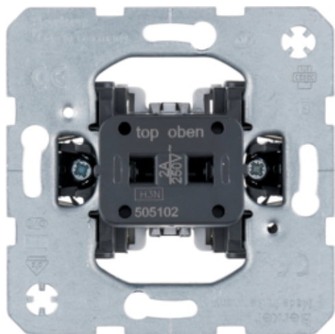
Кнопочний вимикач hotelcard, 1НВ, 2А/250В
