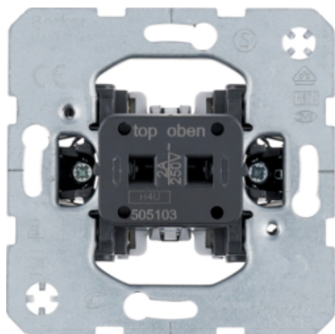
Кнопочний вимикач hotelcard, 2 роздільн.сигнальн.контакти, 2A/250V
