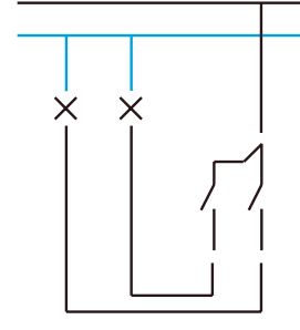
Выключатель двухклавишный
